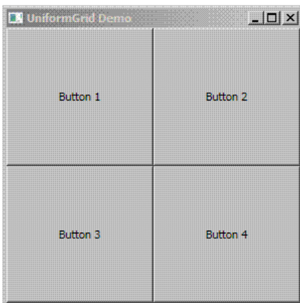
Abbildung 3-7: UniformGrid Beispiel 1
