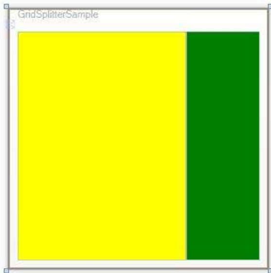
Abbildung 3-3: GridSplitter Demo 2
