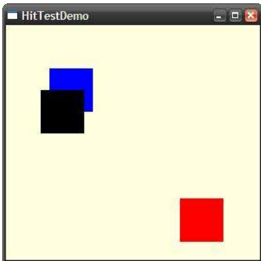
Abbildung 6-3: HitTest Demo 1
