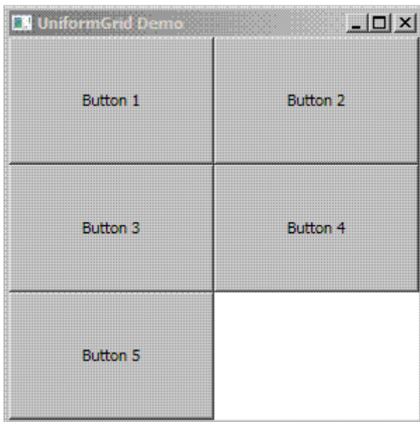
Abbildung 3-9: UniformGrid Beispiel 3
