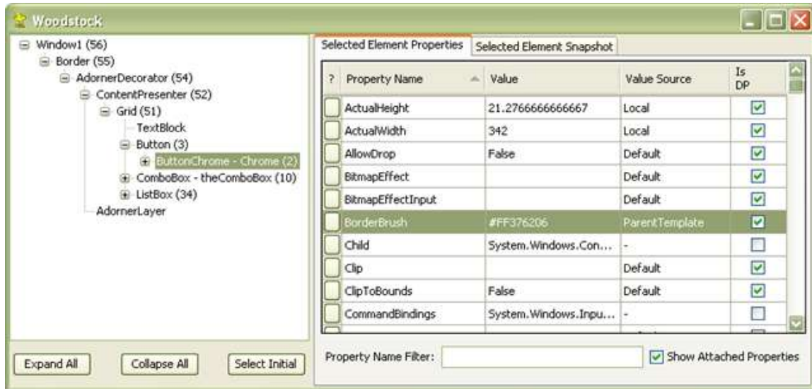
Abbildung 7-2: Screenshot Woodstock
