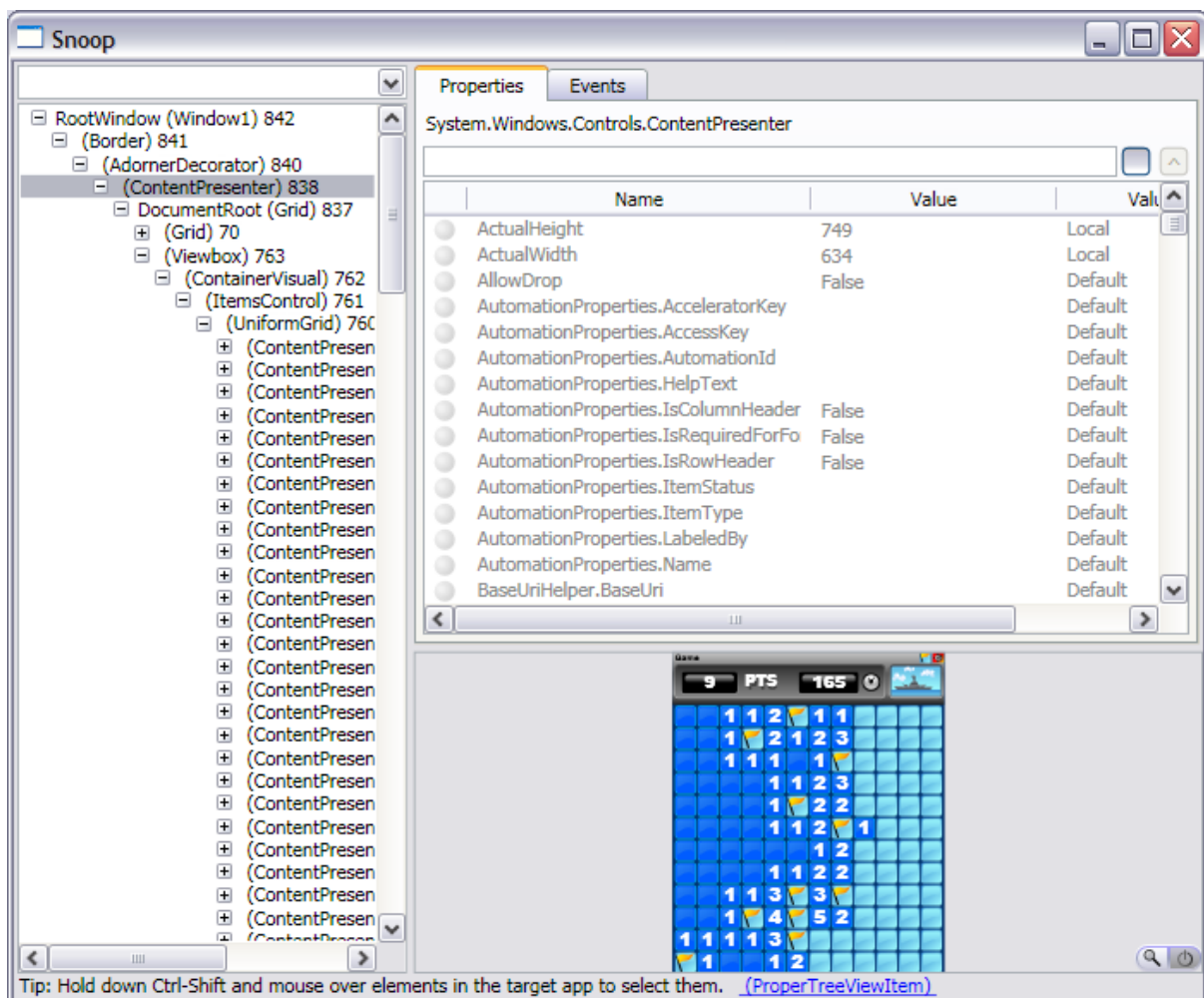
Abbildung 7-1: Screenshot Snoop
