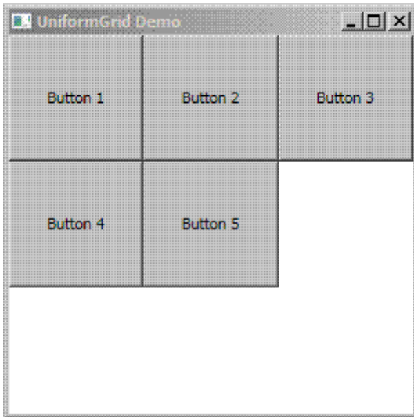
Abbildung 3-8: UniformGrid Beispiel 2
